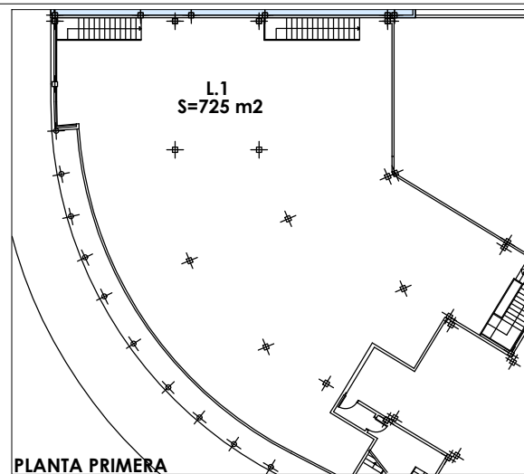
PLANTA PRIMERA
